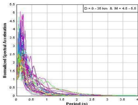
شکل ۵. طیف های پاسخ شتاب افقی نرمال شده به بیشینه شتاب افقی زمین در ۵٪ میرایی برای ایستگاه های مستقر بر ساختگاه های سنگی ایران
