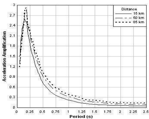
شکل ۱۰. طیف‌های تقویت شتاب افقی نتیجه شده از رابطه تضعیف آمبرسیز و همکاران (۲۰۰۵) در ۰.۵٪ میرایی برای M_s = 5
