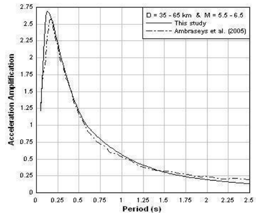
شکل ۱۱. مقایسه طیف طرح افقی حاصل از تحقیقات منطقه‌ای آمبرسیز و همکاران (۲۰۰۵)، با طیف طرح افقی میانگین به‌دست آمده از این تحقیق براساس داده‌های ایران در ۵٪ میرایی.
