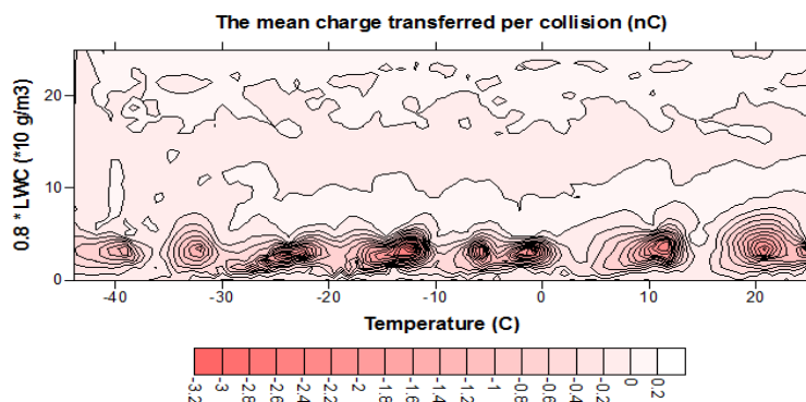
شکل ۲. بار کل تولید شده (nC) در ابر کومه‌ای در شبیه‌سازی ایده آل به صورت تابعی از دما (°C) و محتوی آب مایع موثر درون ابر ( g/m^3 ) با استفاده از روابط پارامتری تاکاهاشی (۱۹۷۸ و ۱۹۸۴). فاصله پربندی nC ۰/۲ ، بیشینه مقدار بار مثبت nC ۰/۰۰۶ و بیشینه مقدار بار منفی nC ۳/۲- است.
