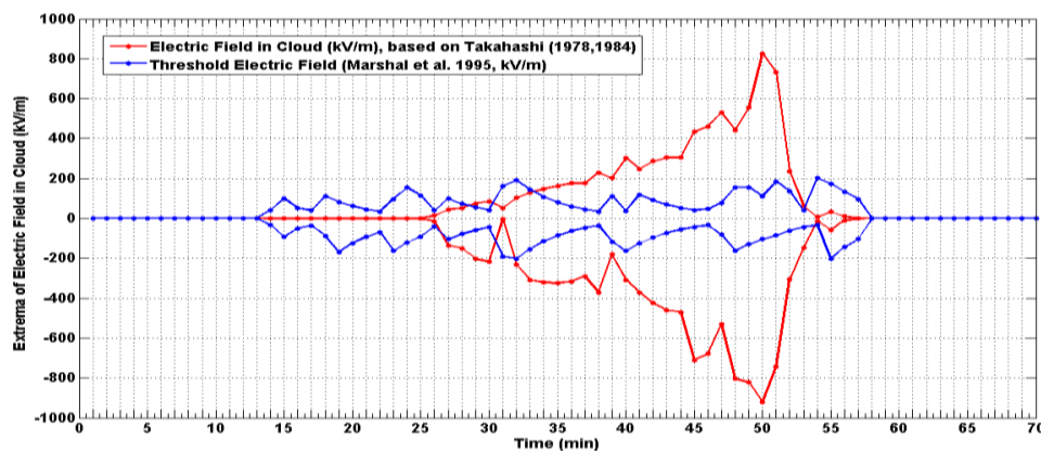
شکل ۵. سری زمانی میدان الکتریکی بار درون ابر در طی ۷۰ دقیقه شبیه‌سازی. خط‌های سرخ‌رنگ مقادیر بیشینه (میدان الکتریکی مثبت) و کمینه (میدان الکتریکی منفی) شبیه‌سازی شده براساس پارامتری تاکاهاشی (۱۹۷۸، ۱۹۸۴) و خط‌های آبی‌رنگ مقادیر آستانه لازم برای شکل‌گیری آذرخش معرفی شده مارشال و همکاران (۱۹۹۵) را نشان می‌دهد.
