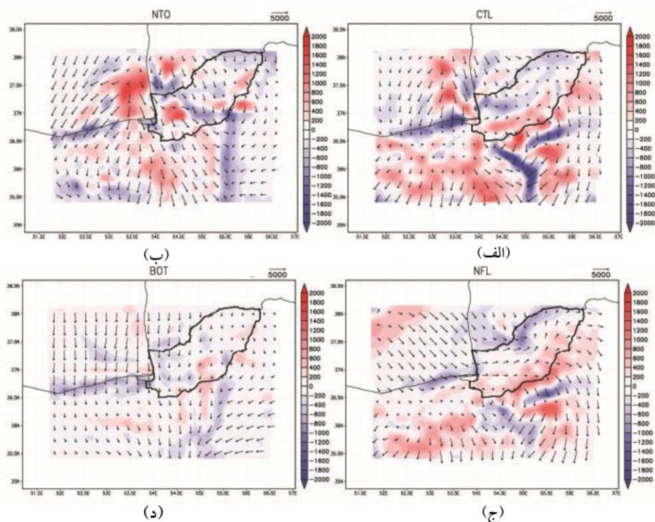
شکل ۵. مانند شکل ۳ ولی برای شار گرمایی افقی در سطح زمین. بردارها، شار افقی گرمایی را برحسب \text{Km/s} و سایه روشن همگرایی (مقادیر منفی) و واگرایی (مقادیر مثبت) شار را بر حسب \text{K/s} نشان می‌دهند.
