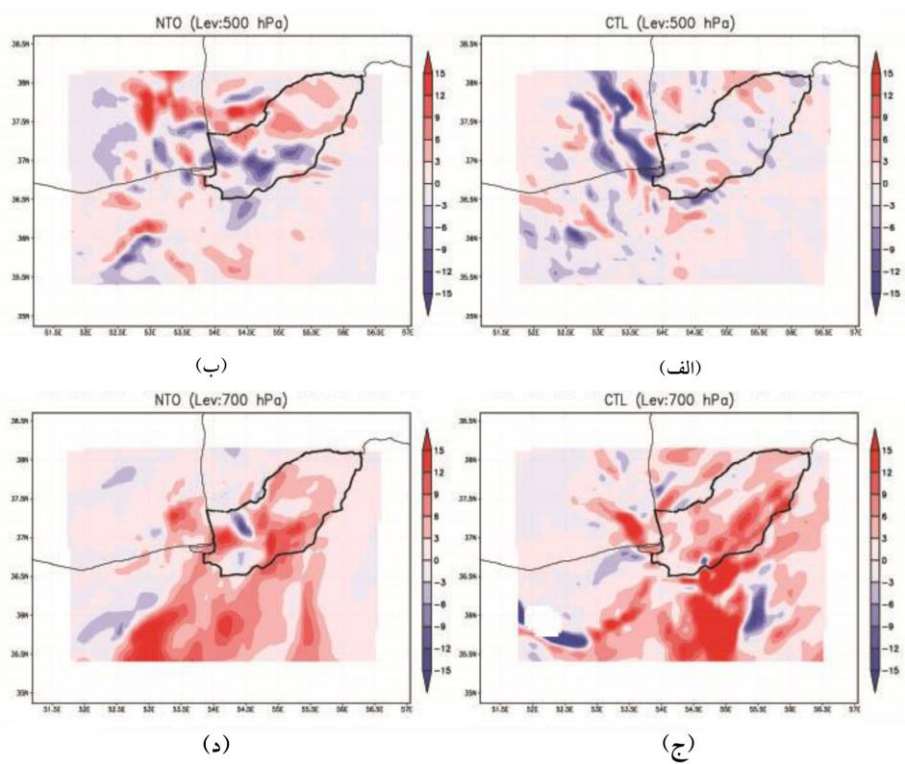
شکل ۳. مقادیر فرارفت دما برحسب کلوین بر شش ساعت در زیر شبکه ۳ در ساعت ۲۱ روز ۱۸ جون ۲۰۱۲ در ترازهای ۵۰۰ هکتوپاسکال (شکل‌های بالا) و ۷۰۰ هکتوپاسکال (شکل‌های پایین). شکل‌های سمت راست برای شبیه‌سازی CTL و شکل‌های سمت چپ برای شبیه‌سازی NTO است.
