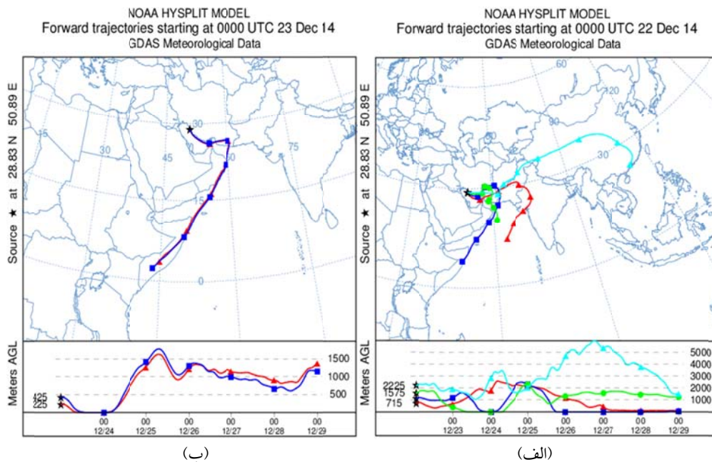
شکل ۹. مسیر انتقال مواد هسته‌ای رها شده از ارتفاعات مختلف، یک هفته بعد از وقوع حادثه در اول دی ۱۳۹۳، مواد پرتوزای رها شده در روز اول و از ارتفاعات ۷۱۵، ۱۰۹۰، ۱۵۷۵ و ۲۲۲۵ متری به ترتیب مسیر مشخص شده با رنگ قرمز، آبی، سبز و فیروزه‌ای در شکل ۹-الف را طی می‌کنند. موادی که در روز دوم از ارتفاعات ۲۲۵ و ۴۲۵ متری رها می‌شوند، به ترتیب مسیری را طی می‌کنند که در شکل ۹-ب با رنگ قرمز و آبی نشان داده شده است.
