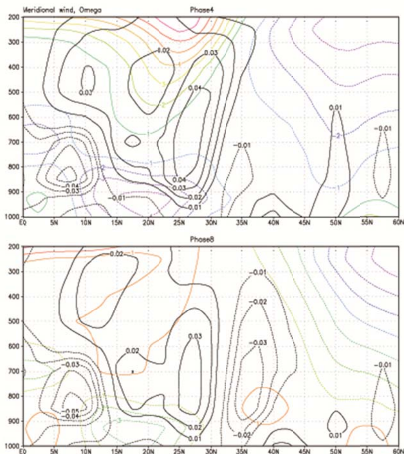
شکل ۶. سطح مقطع قائم میانگین مداری مؤلفه‌های نصف‌النهاری (خطوط رنگی) و قائم (خطوط مشکی) باد از ۲۰ تا ۴۰ درجه شرقی برای فاز ۴ (الف) و فاز ۸ (ب) رخداد MJO. بازه پربندی برای باد نصف‌النهاری ۱ m/s و برای امگا 10^{-1} \text{ s}^{-1} است. مقادیر منفی با خط‌چین نمایش داده شده است.
