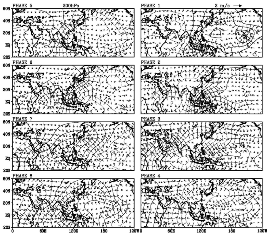
شکل ۲. میانگین بی‌هنجاری پتانسیل سرعت در تراز ۲۰۰ هکتوپاسکال برای هشت فاز مختلف MJO به همراه بی‌هنجاری مؤلفه واگرایی باد از ۲۰ درجه جنوبی تا ۶۰ درجه شمالی و ۰ تا ۲۴۰ درجه طول جغرافیایی. بازه پربندی 1 \times 10^6 \text{ m}^2 \text{ s}^{-1} بوده، مقادیر منفی با خط چین نشان داده شده و خط صفر حذف شده است.
