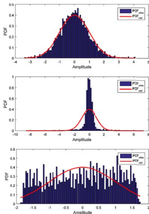
شکل ۲. نویزهای یک‌ساعته ثبت شده در ایستگاه IR1 شبکه ایلپا (چپ) و مقایسه چگالی احتمال محاسبه شده و مشاهده شده برای پنجره نویز به طول یک ساعت (راست). سیگنال بالا با پیروی از توزیع گوسی به‌عنوان نویز مفید وارد مراحل بعدی پردازش می‌شود.
