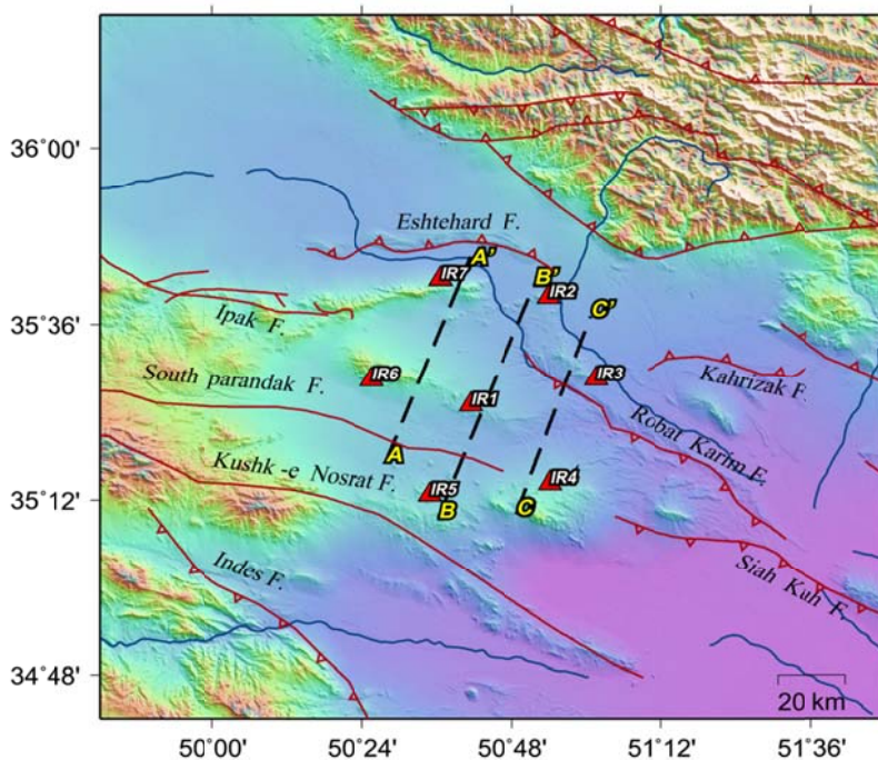
شکل ۱. نقشه موقعیت ایستگاه‌های لرزه‌نگاری درون‌چاهی ایلیا که در سال‌های ۱۳۵۵ تا ۱۳۵۷ ه.ش فعال بوده‌اند. خط‌چین‌ها راستای مقاطع عرضی برآورد سرعت موج برشی را نشان می‌دهند. خطوط قرمز رنگ گسل‌های اصلی منطقه و خطوط آبی مسیر رودخانه‌های اصلی را نشان می‌دهند.
