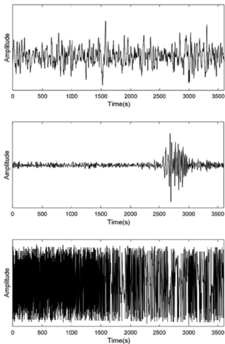
شکل ۲. نویزهای یک‌ساعته ثبت شده در ایستگاه IR1 شبکه ایلپا (چپ) و مقایسه چگالی احتمال محاسبه شده و مشاهده شده برای پنجره نویز به طول یک ساعت (راست). سیگنال بالا با پیروی از توزیع گوسی به‌عنوان نویز مفید وارد مراحل بعدی پردازش می‌شود.
