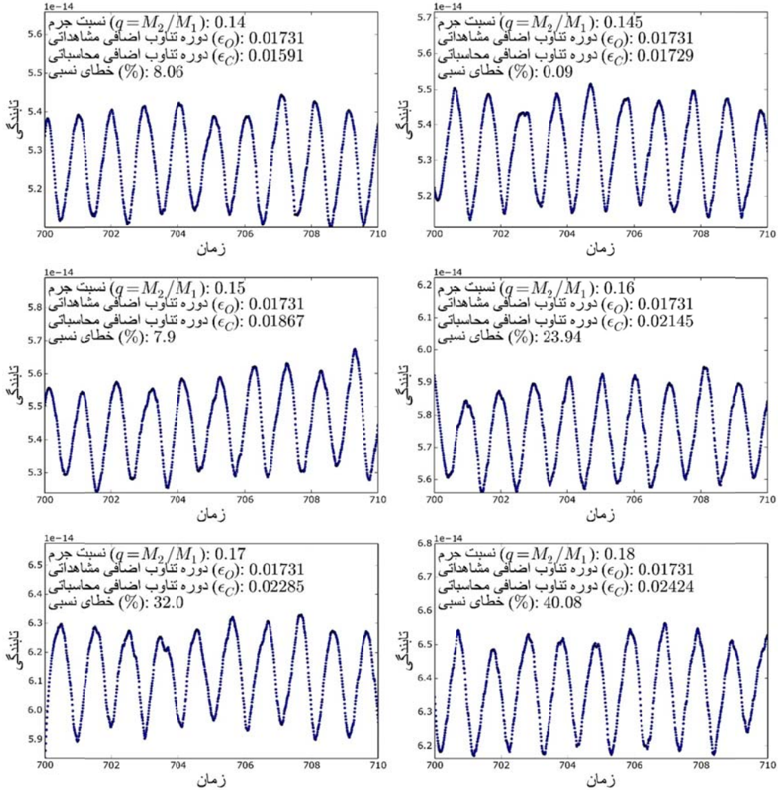
شکل ۵. ظهور برآمدگی‌های متناسب (سوپرهامپ‌ها) در منحنی نوری قرص خارج از مرکز به‌ازای مقادیر مختلف نسبت جرم.
