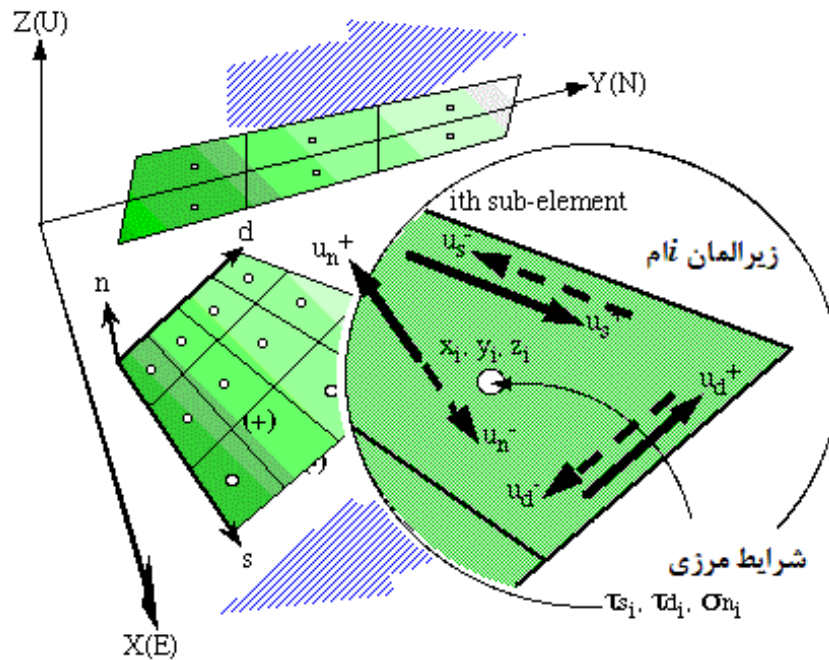
شکل ۲. الگوریتم المان مرزی سه بعدی (گمبرگ و ایس، ۱۹۹۴).
