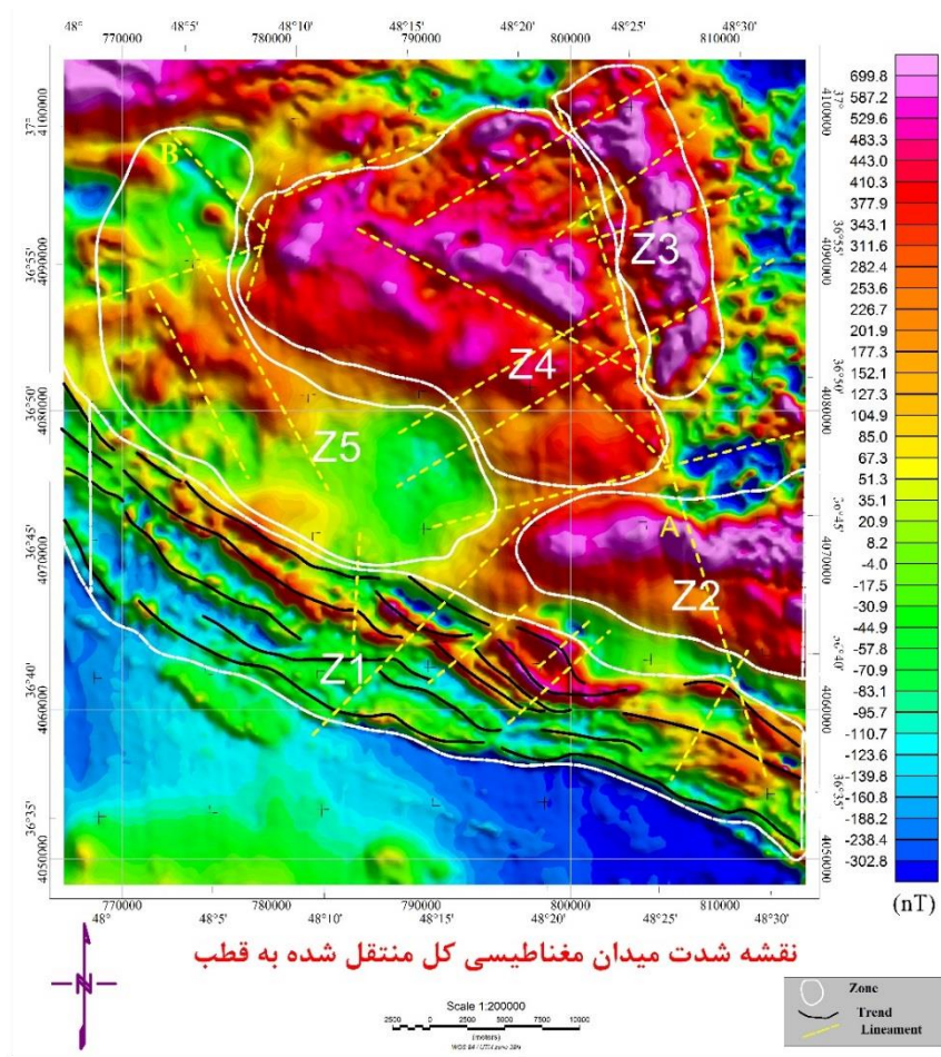
شکل ۵. نقشه مغناطیس هوابرد برگردان به قطب گستره فروافتادگی زنجان. خطوط ممتد مشکی نشان‌دهنده روندهای موجود در منطقه و خط‌چین زردرنگ نمایانگر خطواره‌های شناسایی شده است. همچنین نواحی مختلف با خطوط سفید مشخص شده‌اند. خطواره A یک گسل طولانی شمال-جنوب خاور را نشان می‌دهد که در نقشه زمین‌شناسی منطقه (شکل ۴) مشخص شده است. همچنین خطواره B احتمال وجود گسلی عمیق را نشان می‌دهد که پس از اعمال فیلتر زاویه تیلت گرادیان افقی مشخص شده است و در نقشه زمین‌شناسی منطقه ترسیم نشده است.
