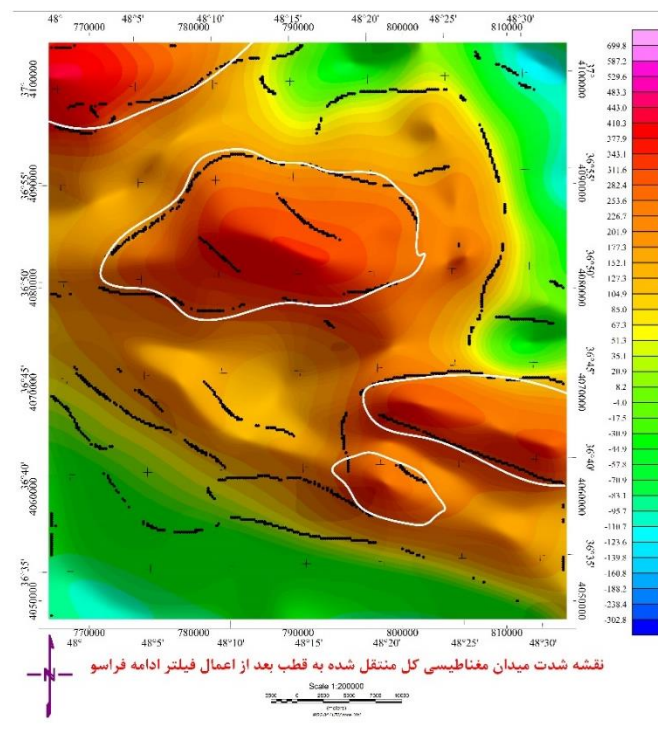
شکل ۸. نقاط سیاه‌رنگ، مکان‌هایی از نقشه مغناطیس هوابرد برگردان به قطب منطقه پس از اعمال فیلتر ادامه فراسو به اندازه ۳ کیلومتر است که در آن زاویه تیلت گرادیان افقی بیشینه است. خطوط سفید مقادیر بیشینه‌ای که مرز پی‌سنگ را مشخص می‌کند، نشان می‌دهد.
