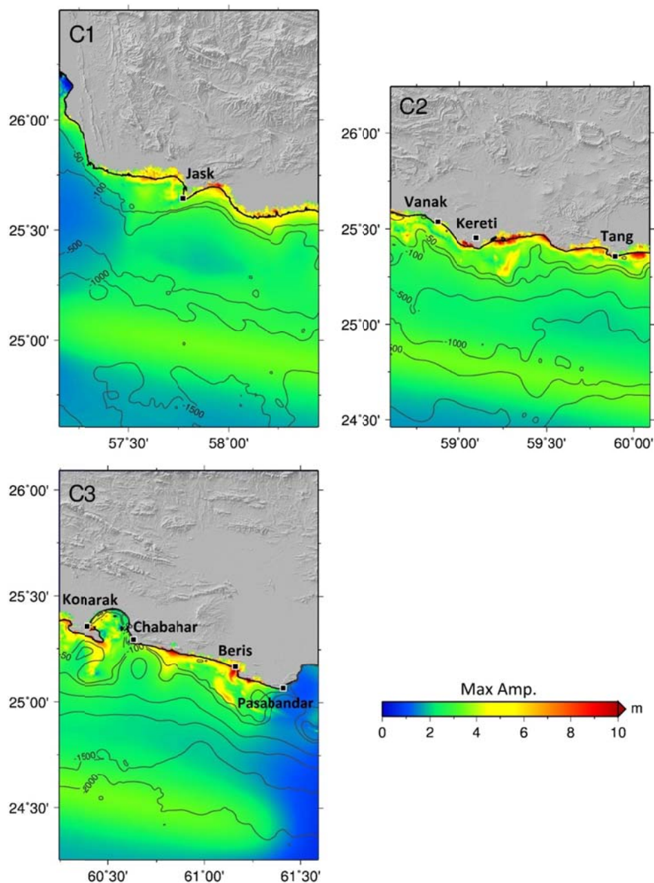
شکل ۷. نقشه بیشینه ارتفاع موج شبیه‌سازی شده برای چشمه زمین‌لرزه در مناطق C1، C2 و C3. کتورها نشان‌دهنده عمق آب بر حسب متر هستند.
