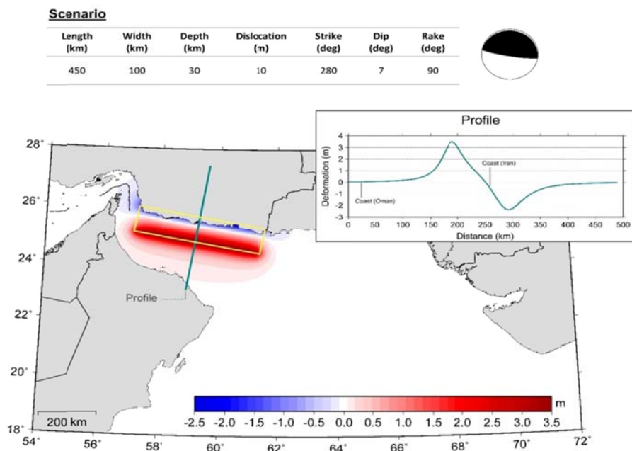
شکل ۱. مشخصات سناریوی به کار گرفته شده برای شبیه سازی سونامی و میدان دگرشکلی محاسبه شده برای آن که به عنوان شرایط اولیه در شبیه سازی COMCOT استفاده شده است (رشیدی و همکاران، ۱۳۹۷). نواحی قرمز رنگ بالا آمدگی و نواحی آبی رنگ فروافتادگی را بر حسب متر نشان می دهند. تصویر صفحه گسل بر روی سطح زمین با خط زرد رنگ مشخص می باشد.
